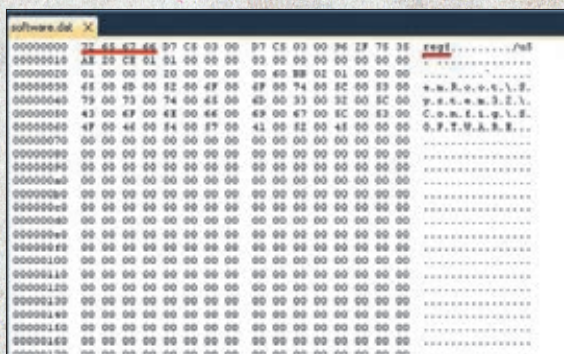
Авот и сигнатура «regf»...
