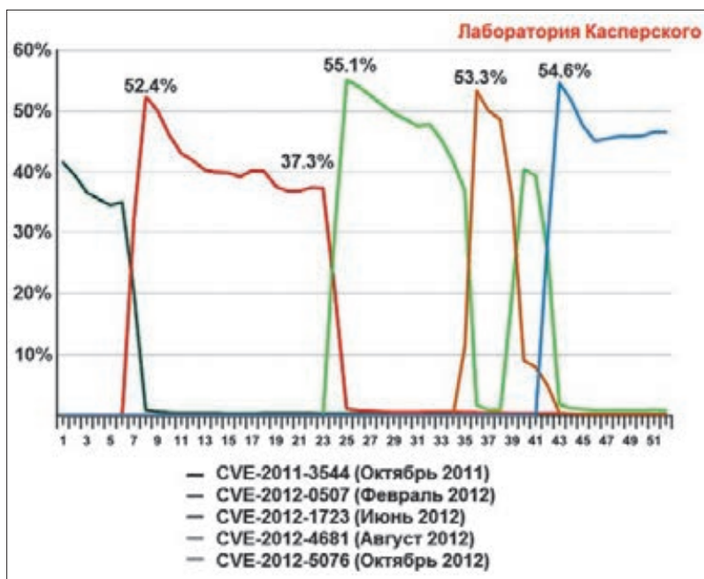
Рис. 2. Статистика использования уязвимостей Java
