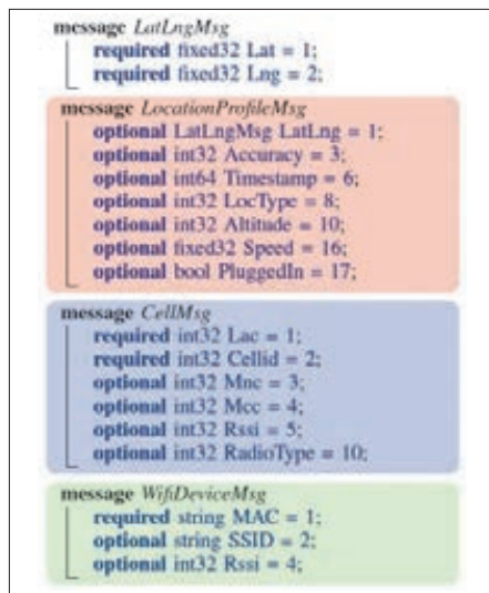
Рис. 1. Шаблон полезной нагрузки для запросов и ответов по протоколу Protocol Buffers
