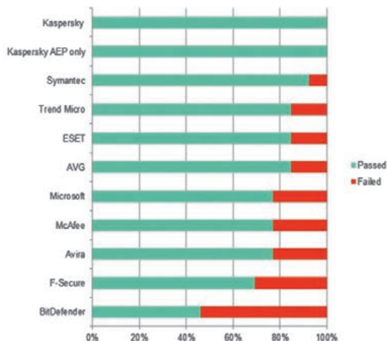
Результаты тестирования технологии AEP лабораторией MRG Effitas
